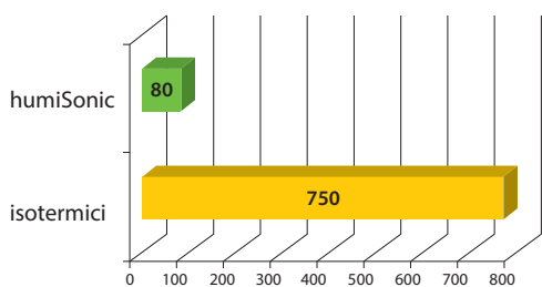
Confronto del consumo elettrico tra humiSonic e gli umidificatori a vapore (Watt per kg/h di acqua evaporata).
