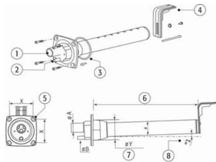
Fig. 4.a - Montage der Dampfzweiger
