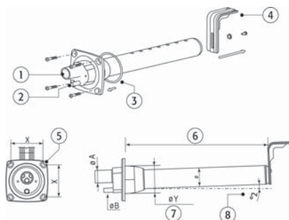
Fig. 4.a - Montage des distributeurs
