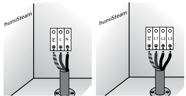
Fig. 4.c (vista interna da máquina, vão elétrico)
