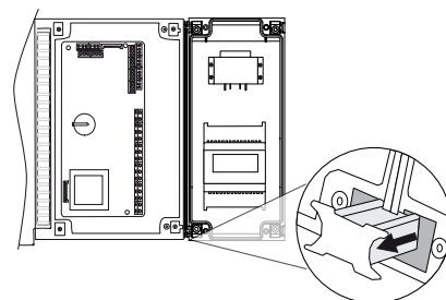
exemple avec UltraCella + module Ultra EVD
