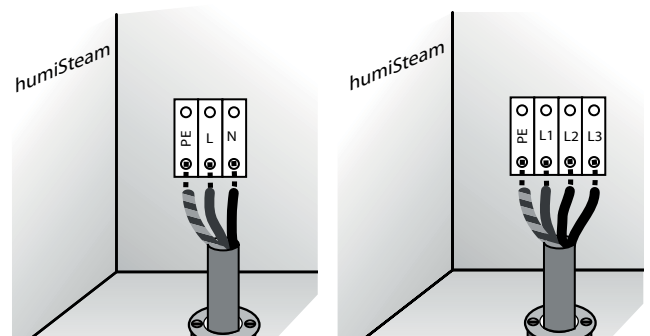
Fig. 4.c (Innenansicht, Elektroteil)
