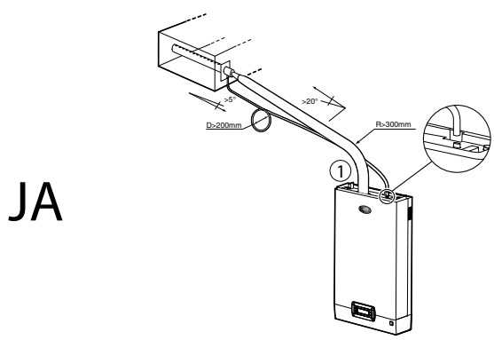
Modelle UE001...UE025 (1): Verbindung mit Zulaufwanne
