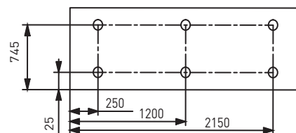
Расположение виброопор моделей 039...096-W3-AT
