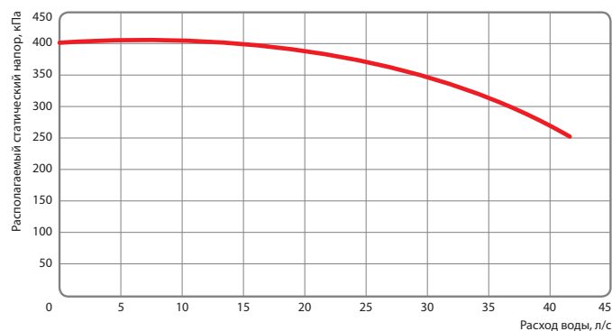
Характеристика С (KSM 1C и KSM2C)
