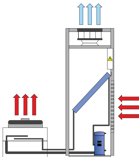
Прецизионный кондиционер для работы с выносным конденсатором и выхлопом вверх
