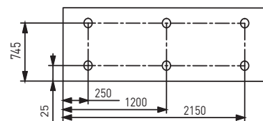
Расположение виброопор моделей 079-190
