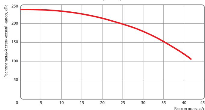
Характеристика D (KSM 1D и KSM2D)
