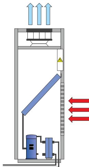
Прецизионный кондиционер с конденсатором водяного охлаждения для работы с драйкулером и выхлопом вверх
