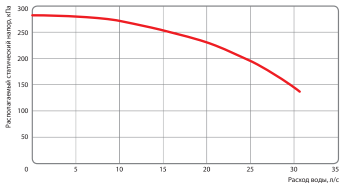
Характеристика А (KSM 1A и KSM2A)
