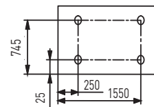
Расположение виброопор моделей 039-072
