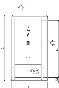
Вид „А-А”
