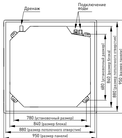
Типоразмеры KF-FCU-53-CT – KF-FCU-100-CT
