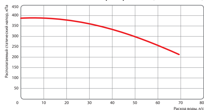
Характеристика F (KSM 1F и KSM2F)
