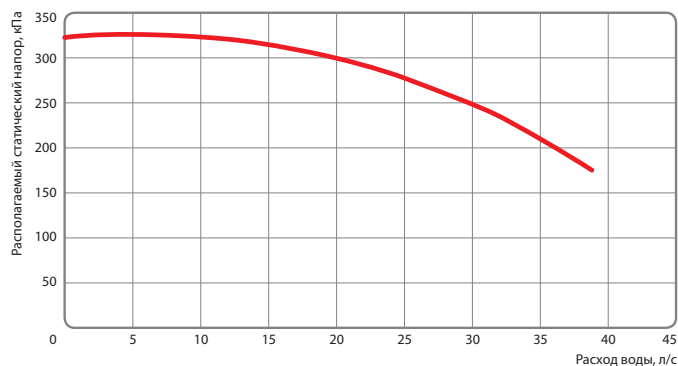
Характеристика В (KSM 1B и KSM2B)
