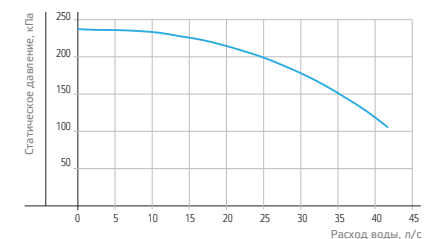
Характеристика F (NST 1F и NST 2F)
