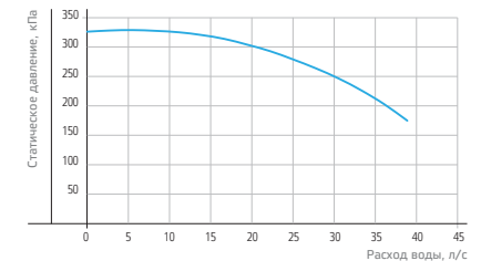
Характеристика D (NST 1D и NST 2D)
