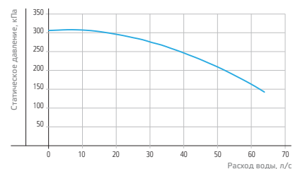
Характеристика E (NST 1E и NST 2E)
