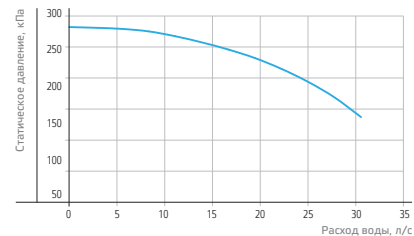
Характеристика С (NST 1С и NST 2С)
