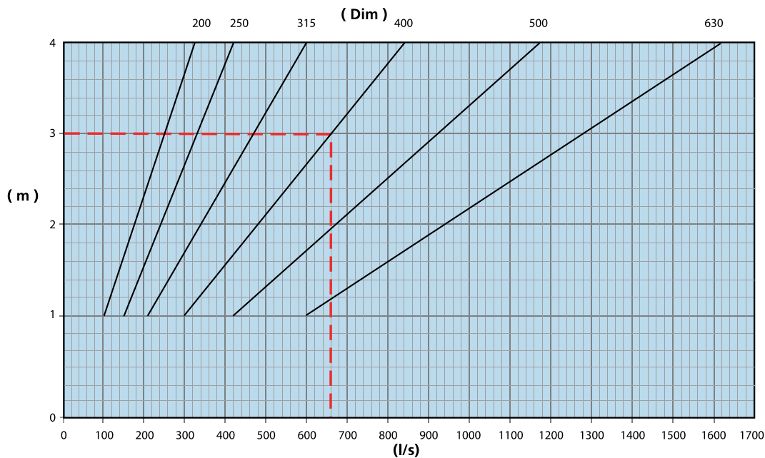
Диаграмма 1. Глубина проникновения струи вниз (м), обогрев, \Delta T +5 \text{ K}
