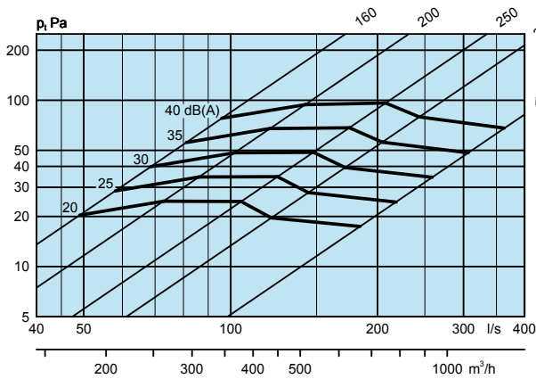
LPA 160, 200, 250, 315, 400, Вытяжка
