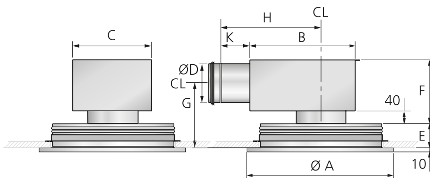
Рис. 3. LPA + ALS
