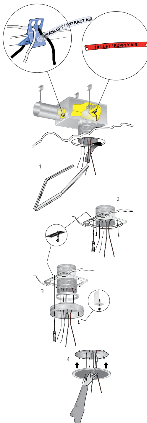
Рис. 1. Монтаж
