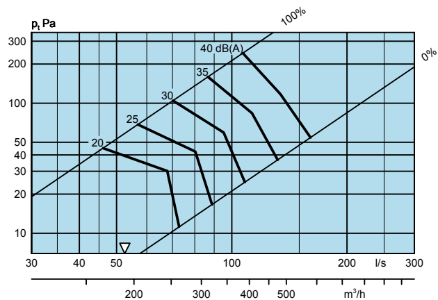
ALG 500-100 + TRG-B Ø200, Вытяжка
