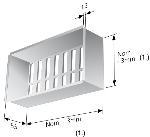
Рис. 4. Крепежная рама со вставной заслонкой FHB
