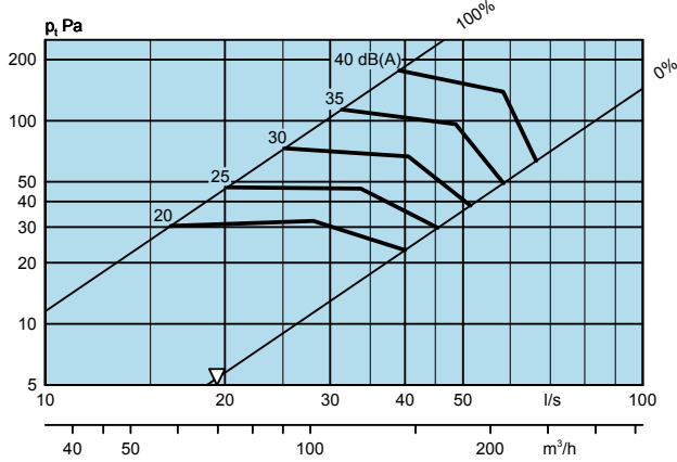
ALG 200-100 + TRG-B Ø125, Вытяжка
