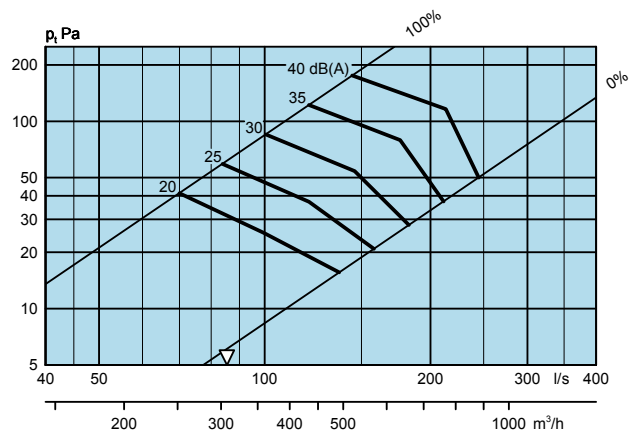
ALG 500-150 + TRG-B Ø250, Вытяжка
