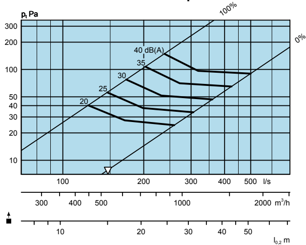
ALG 600-200 + TRG-B Ø315, Приток
