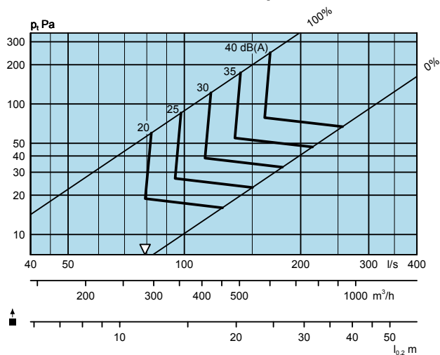
ALG 500-150 + TRG-B Ø250, Приток
