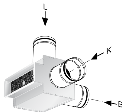
Рис. 5. Варианты подсоединения для TRG
