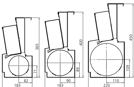
Рис. 12. Вид сбоку Ø125, Ø160 и Ø200
