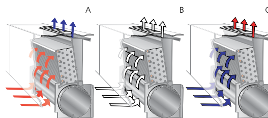
Рис.1. Рабочие режимы: A = охлаждение, B = только вентиляция, C = обогрев (вода или электричество)
