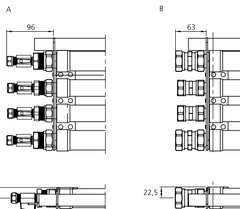
Рис. 14. Соединительные детали A=Конец трубы, B=Муфта трубопровода
