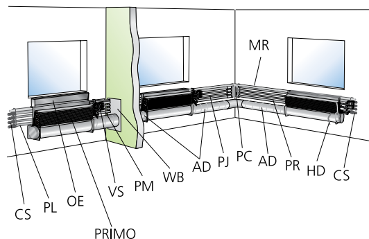
Рис. 10. Сборная схема принадлежностей
