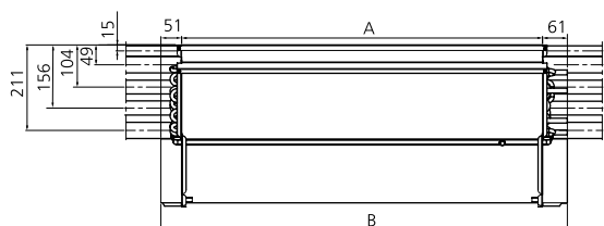
Рис. 11. Вид спереди (фронт) A=Выдвижное устройство, длина (изнутри) всегда 110мм; B=Длина
