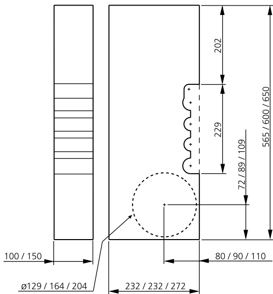
Рис. 17. Стеновой блок WB
