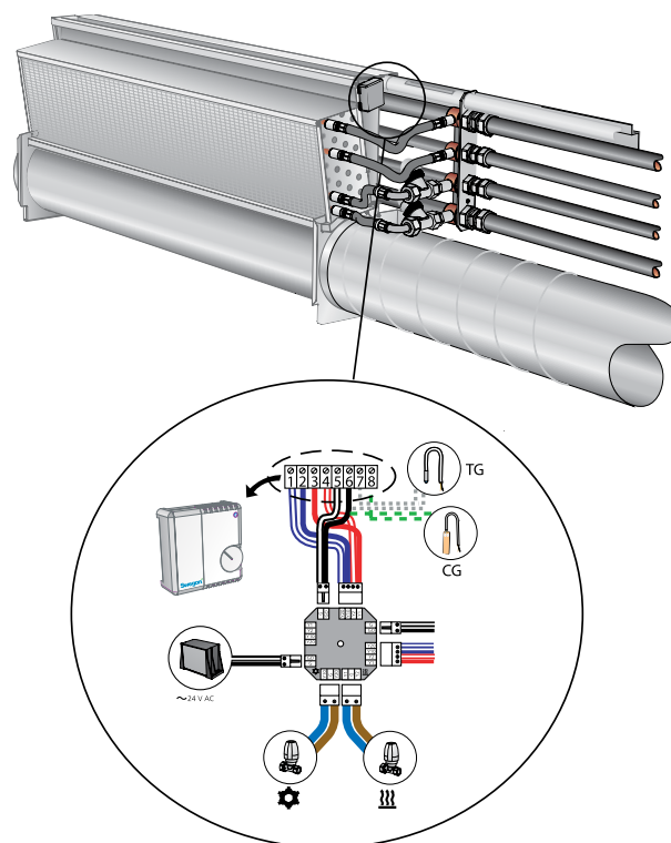
Рис. 18. Оборудование автоматики LUNA Для подключения электрокалорифера смотрите отдельную инструкцию на нашем сайте
