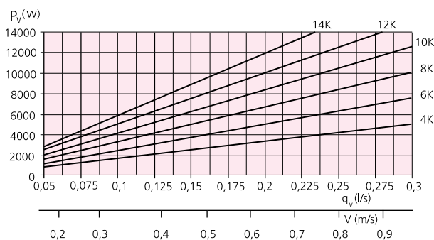
Диаграмма 5. Расход воды - теплопроизводительность, ветвь
