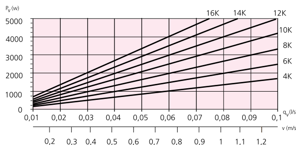
Диаграмма 5. Расход воды - теплопроизводительность, ветвь
