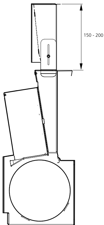
Рис. 16. Выдвижное устройство
