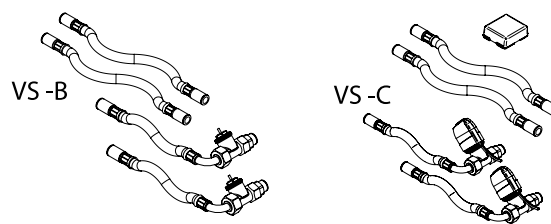
Рис. 7. Набор клапанов VS
