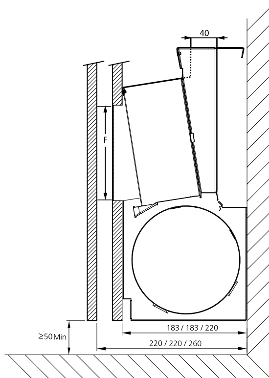
Рис. 15. Пространство для воздуха из помещения Min. расстояние от пола до декоративной обшивки либо до открытия для поступления воздуха из помещения в передней панели обшивки
