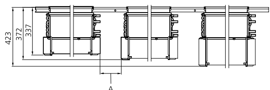
Рис. 13. Монтажная зона A=Min. монтажное расстояние 200 мм
