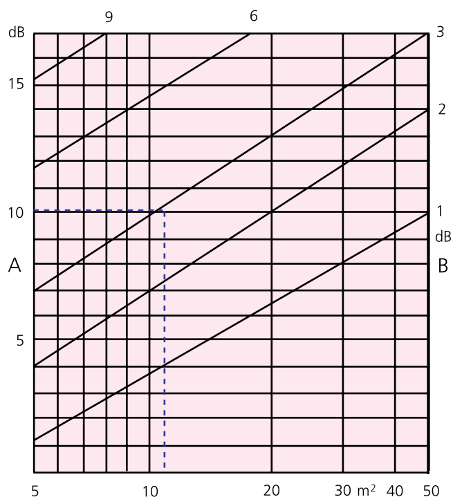
Диаграмма 6. К-т глушения
