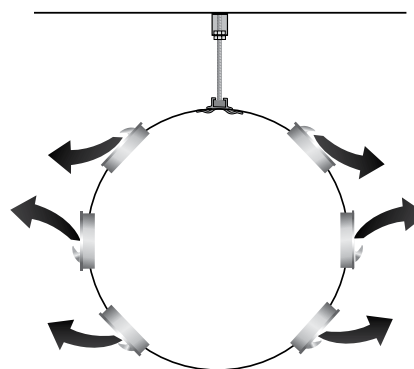
Рис. 5. 2-стороннее распределение, длинная струя. Оба верхних ряда дисков повернуты вниз
