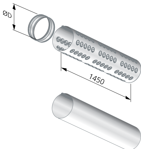
Рис. 7. IBIS и IBIS D*) (Размер одной секции) *) До диаметра 400 включительно
