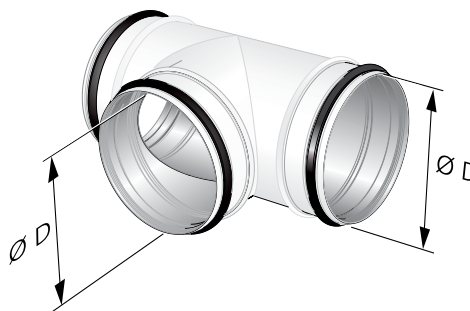
Рис. 10. IBIS T*) *) До диаметра 400 включительно
