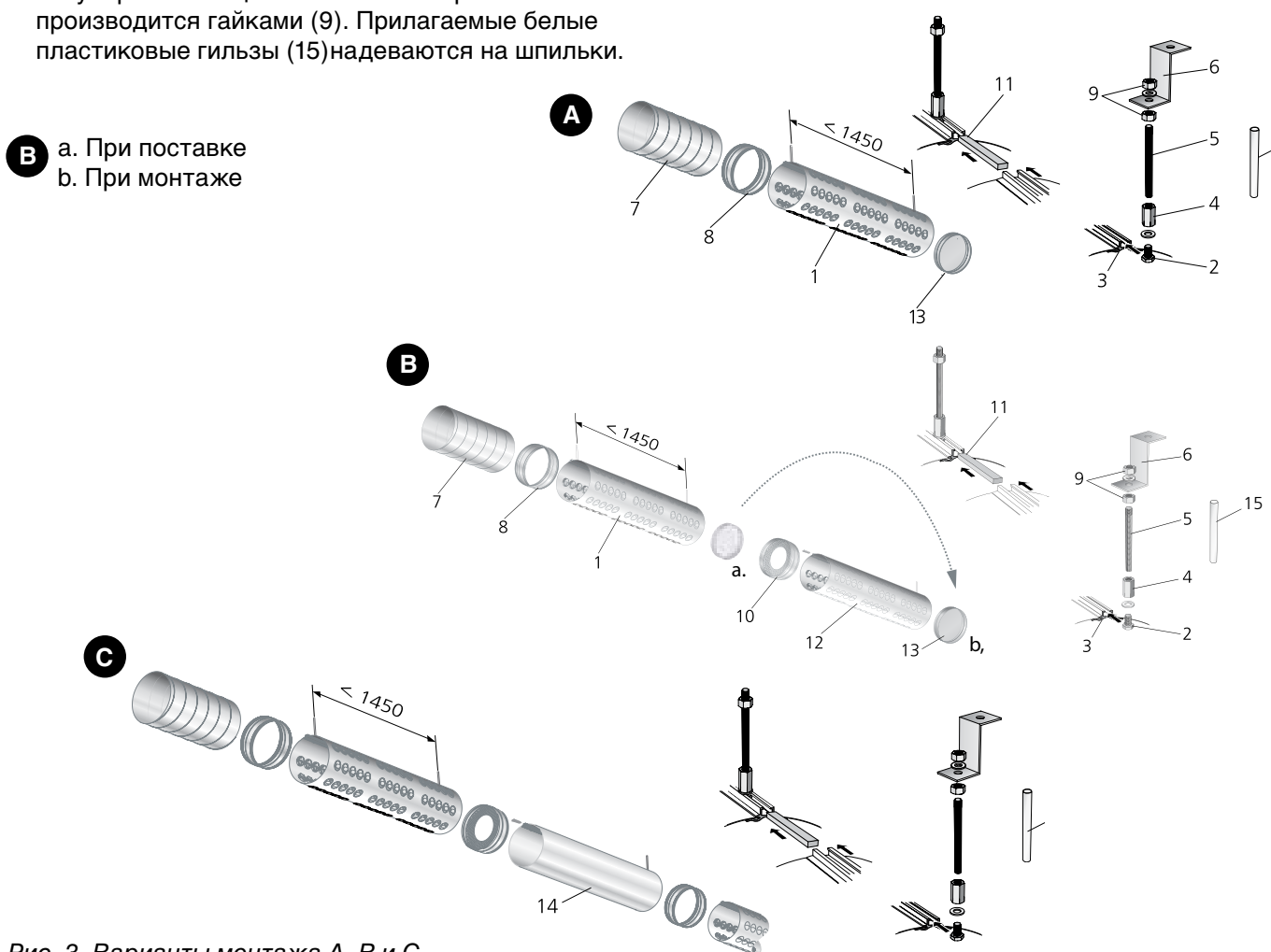
Рис. 3. Варианты монтажа А, В и С
