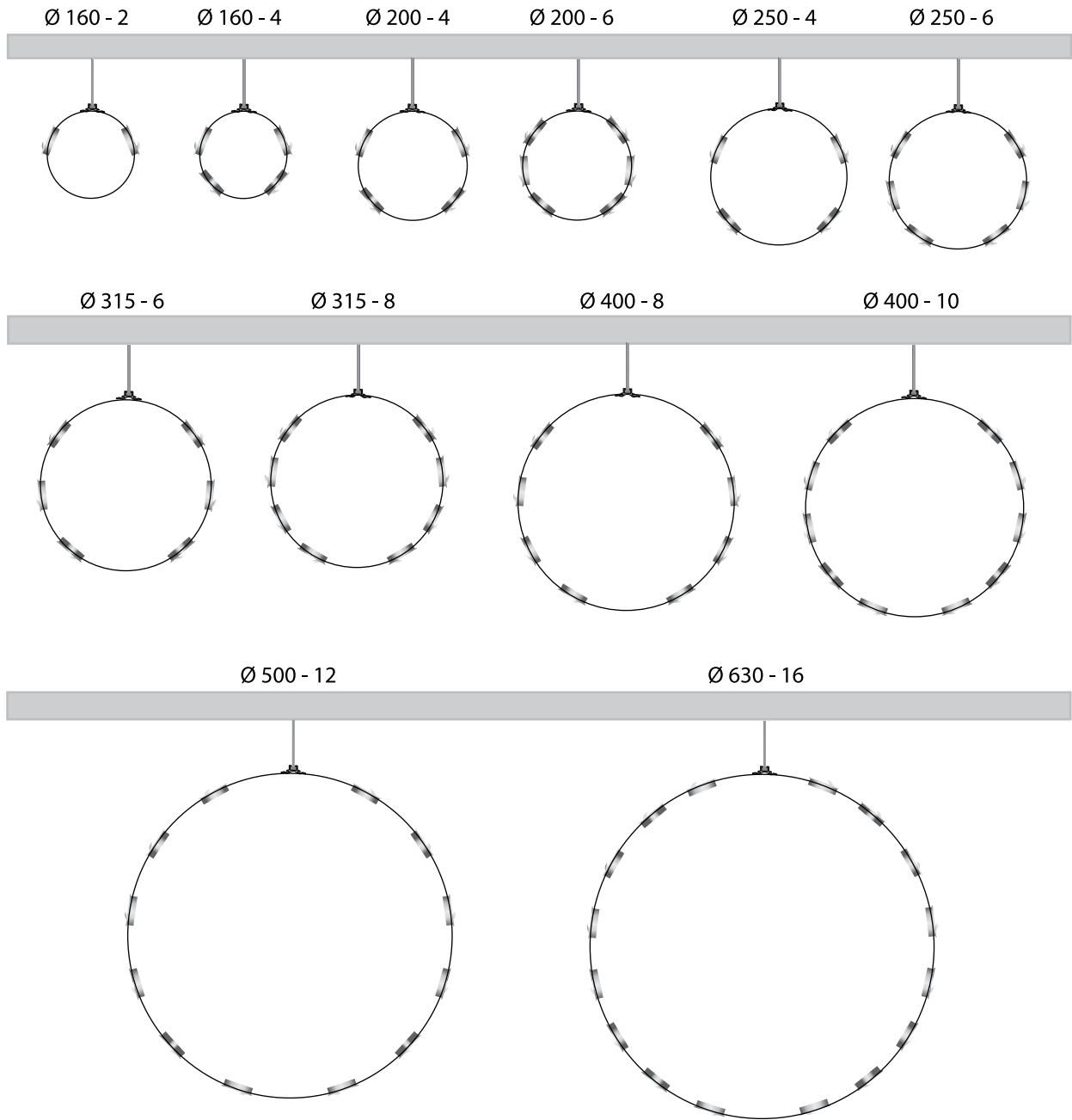
Рис. 11. Расположение дисков
