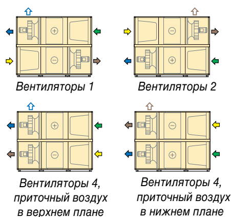
Левое исполнение
