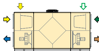
Левое исполнение
