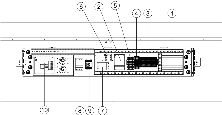
Рис. 2 Электрические компоненты
