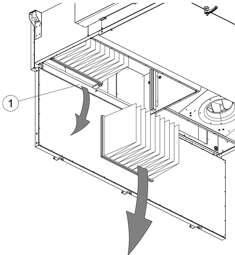
Рис. 5 Замена фильтров
