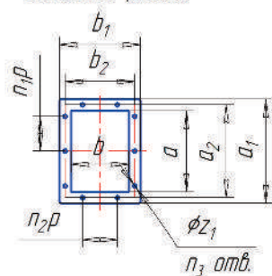
Выходной фланец
