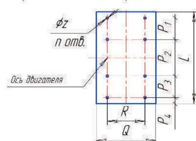
Крепление вентилятора БЕЗ СТОЙКИ
